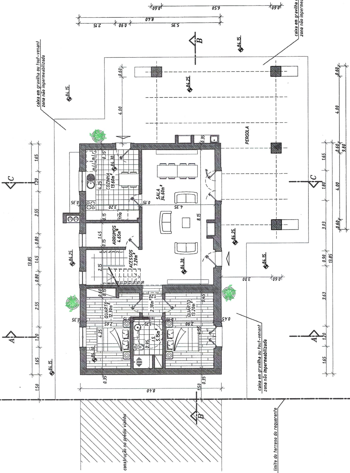
PLANTA DO RÉS DO CHÃO Área Bruta - 116,35m 2
